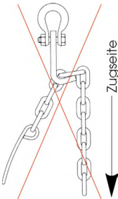
POGREŠNO KAČENJE LANCA
